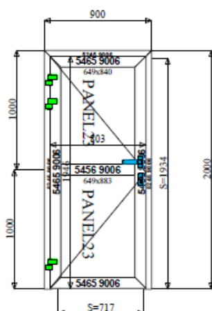
Poz. 2 PE50 - Drzwi otwierane na zewnątrz (B=900, H=2 000) Klamka FP207X8 INOX+Zamek MV+Brak puszki do zaczepu
