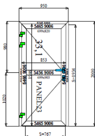
Poz. 1 PE50 - Drzwi otwierane na zewnątrz (B=950, H=2 000) Klamka FP207X8 INOX+Zamek MV+Brak puszki do zaczepu
